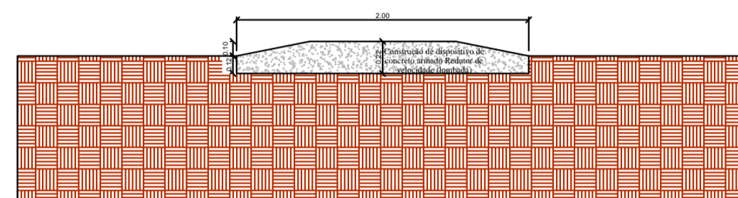
Avenida do Contorno entre Alameda Garcia e Rua Quatro Comprimento da Lombada = 8.20 metros Largura da Lombada = 2 metros Área = 16.40 m 2
