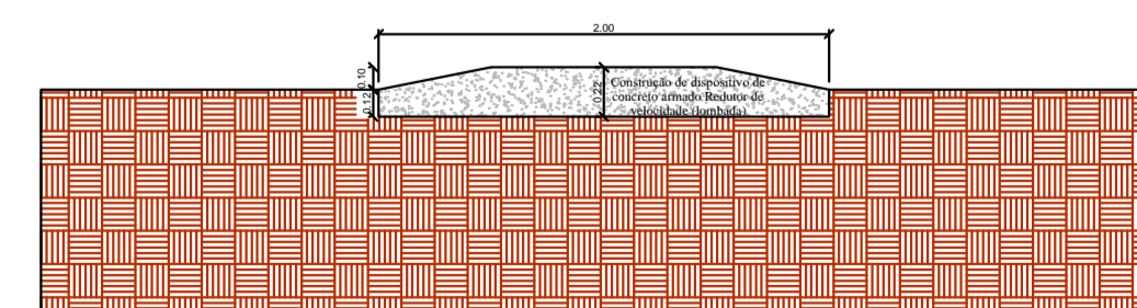
Rua Vinte e Quatro entre avenida Um e Avenida Um A Comprimento da Lombada = 8.20 metros Largura da Lombada = 2 metros Área = 16.40 m 2
