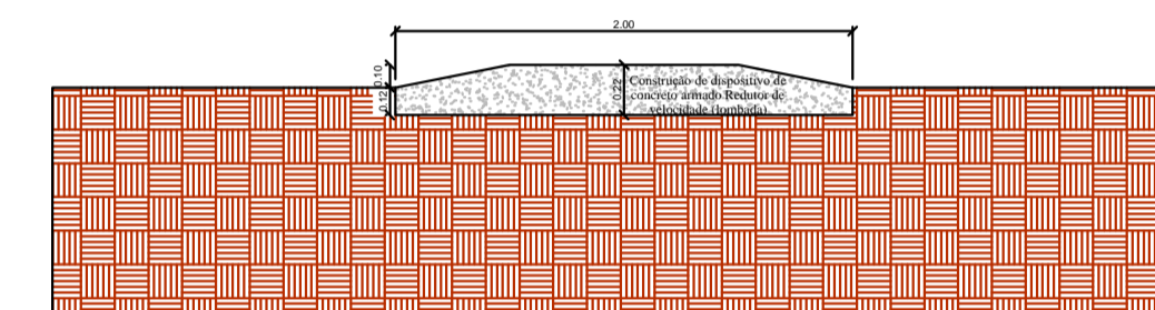
Rua Prefeito Jerônimo Donizete da Silva entre rua Vereador Pedro Crispim e Rua Vereador Vicente Braga Comprimento da Lombada = 8.20 metros Largura da Lombada = 2 metros Área = 16.40 m 2
