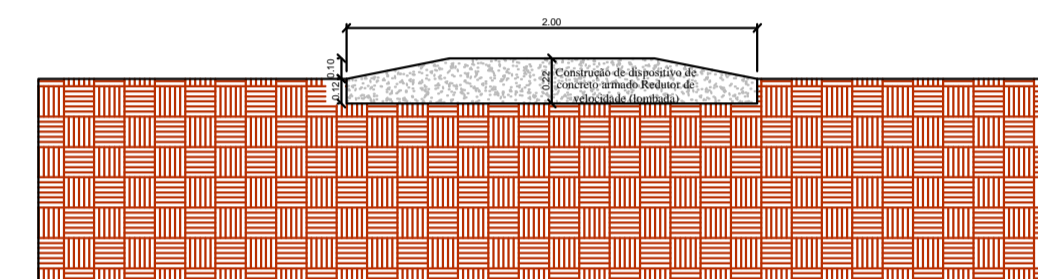
Rua Prefeito Gilberto Queiroz entre avenida João Batista e avenida Vereador Evaristo Moura Soares Comprimento da Lombada = 8.20 metros Largura da Lombada = 2 metros Área = 16.40 m 2
