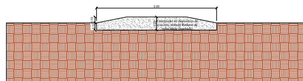
Avenida Vinte e Três entre rua Dezesesseis e rua Dezoito Comprimento da Lombada = 8.20 metros Largura da Lombada = 2 metros Área = 16.40 m 2
