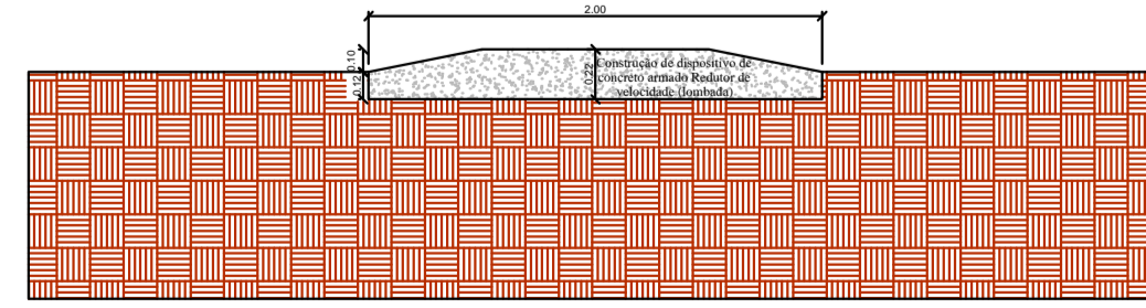
Rua Dezoito entre avenida Onze A e avenida Treze A Comprimento da Lombada = 8.20 metros Largura da Lombada = 2 metros Área = 16.40 m 2
